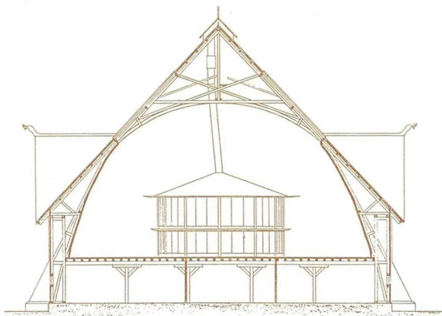
Konstruktionsritning, Biologiska Museet. Arkitekt Agi Lindegren.
